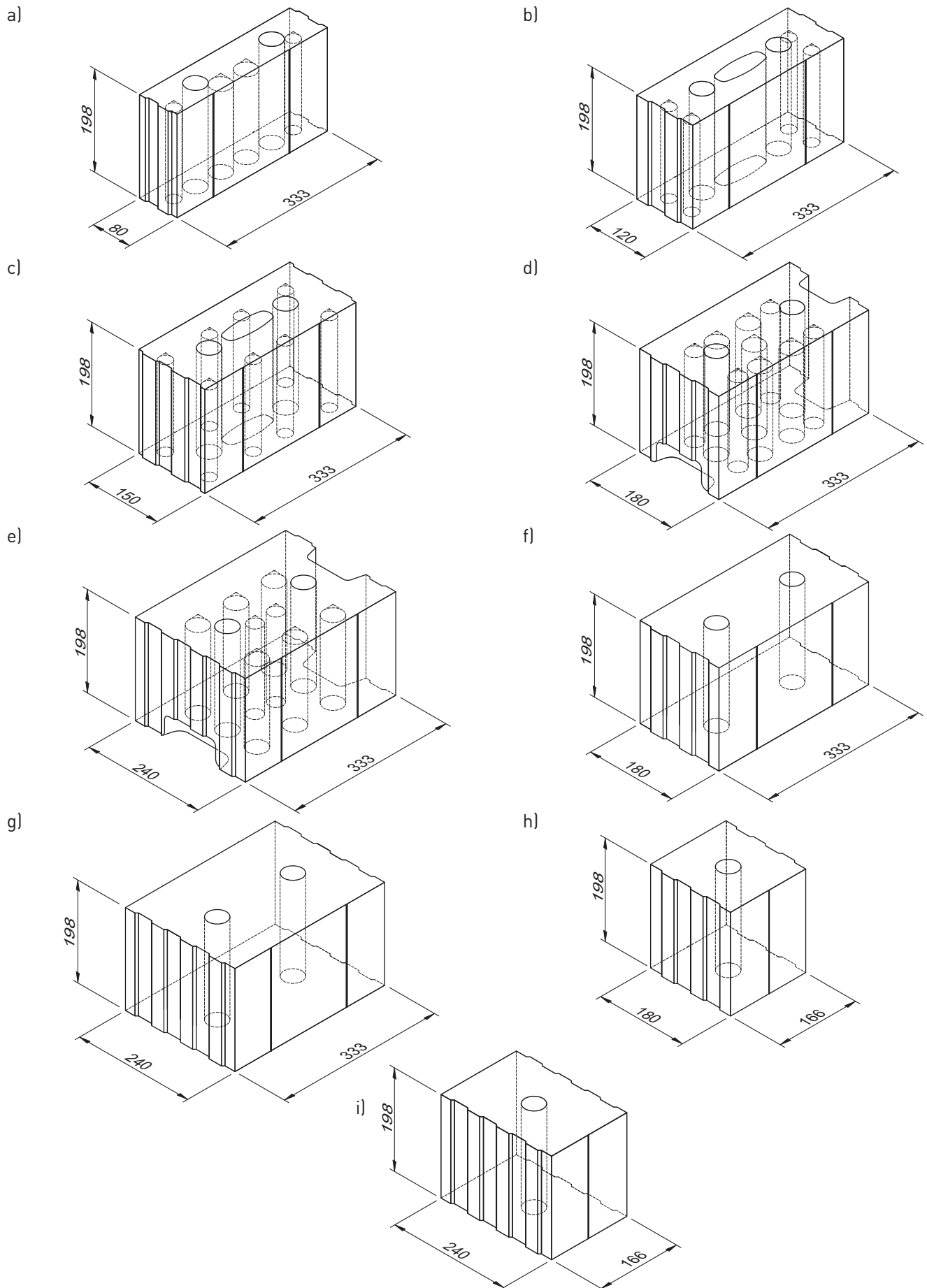
Rys. 2.1. Bloki serii SILKA E: a) SILKA E8, b) SILKA E12, c) SILKA E15, d) SILKA E18, e) SILKA E24, f) SILKA E18S, g) SILKA E24S, h) SILKA 1/2E18, i) SILKA 1/2E24.
